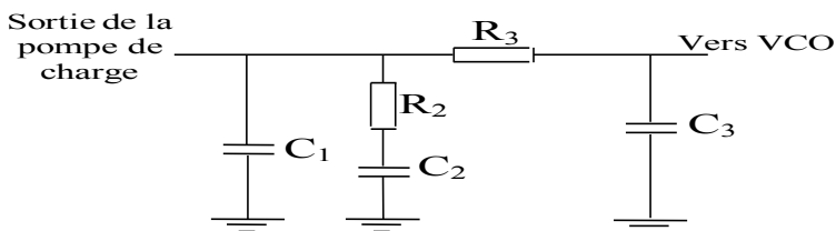
Figure 2 : Filtre passe-bas 3ème ordre
