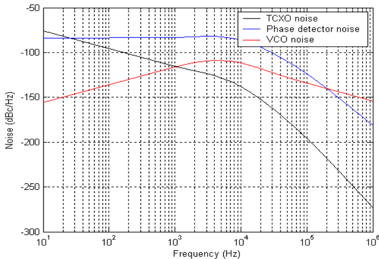
Figure 6 : Contribution des Bruits de TCXO, VCO et détecteur de phase
