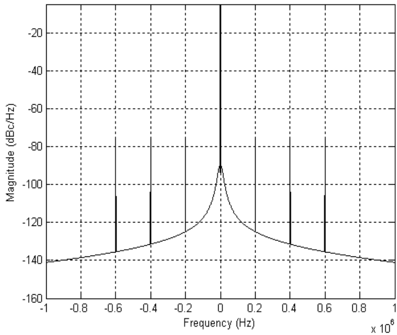
Figure 10 : Spectre de sortie de la PLL
