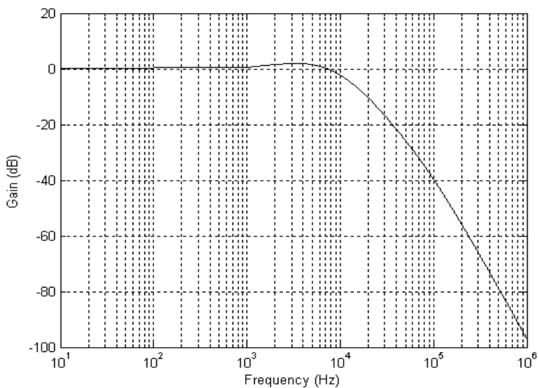
Figure 5 : Réponse de la boucle fermée
