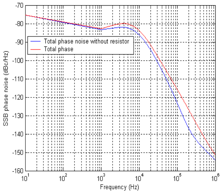
Figure 8 : Bruit de phase avec et sans le bruit des r sistances
