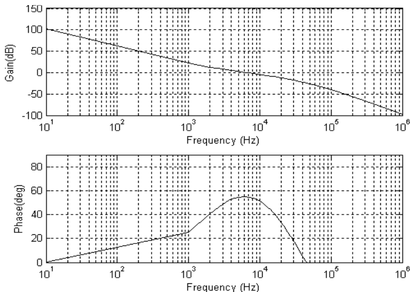
Figure 4 : Réponses de la boucle ouverte
