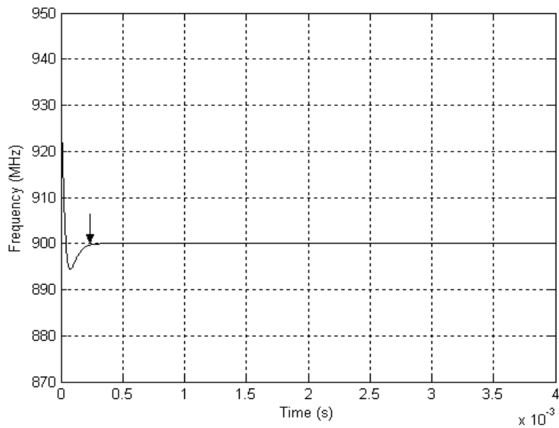
Figure 11 : Réponse temporelle de la PLL
