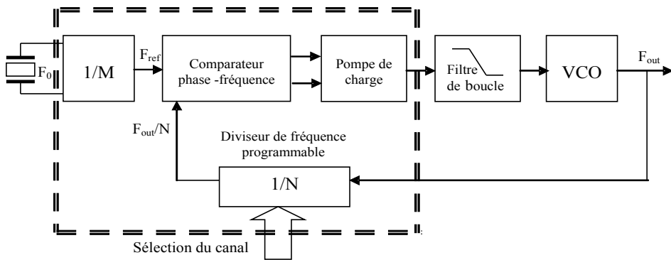
Figure 1 : Synthétiseur de fréquence classique à base de PLL
