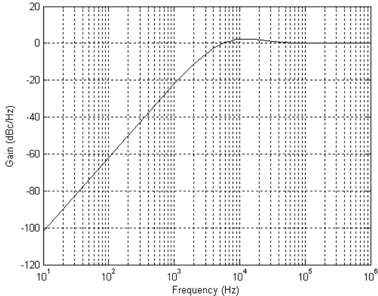
Figure 9 : Réponse d'erreur de la boucle
