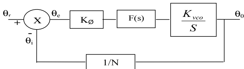
Figure 3 : Modèle linéaire de la PLL
