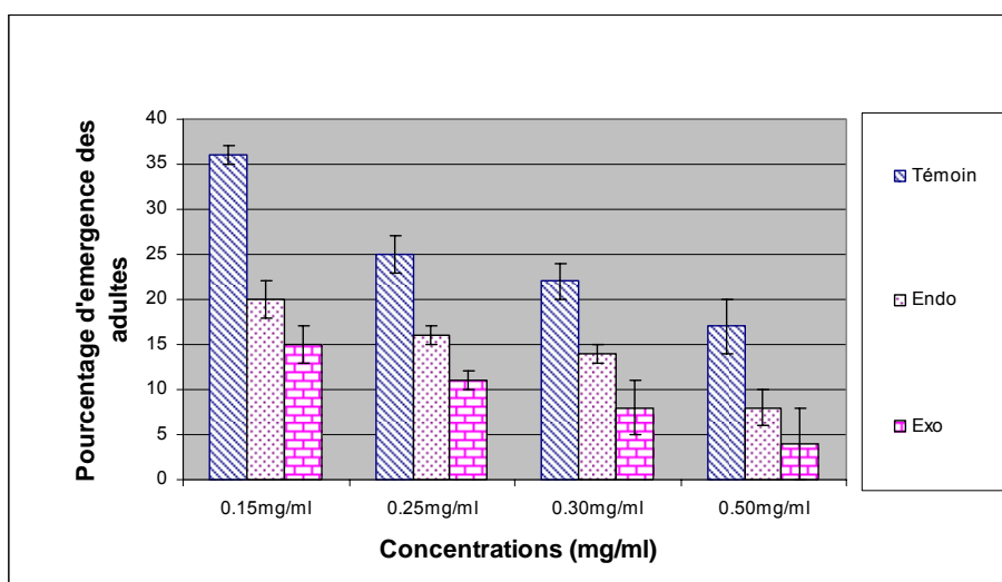
Figure 3: Effet des toxines de la souche de Bt A9 sur l'émergence des adultes de C. capitata (ENDO : endotoxines ; EXO : exotoxines)
