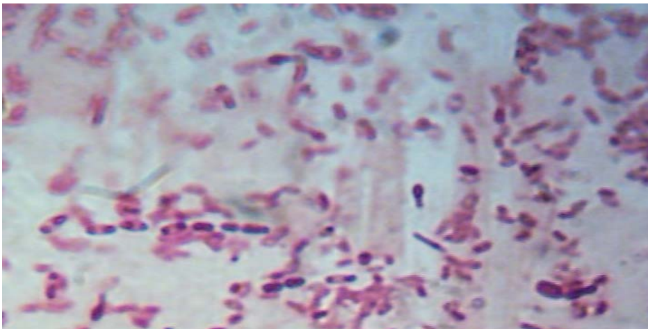
Figure 1 : Photo de la culture sporulée de la souche de Bacillus thuringiensis (Bt A9) avec le corps d'inclusion parasporal (P) (G x 1500)
