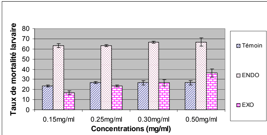
Figure 2 : Effet des toxines de la souche de Bt A9 sur le taux de mortalité larvaire de C. capitata (ENDO : endotoxines ; EXO : exotoxines)
