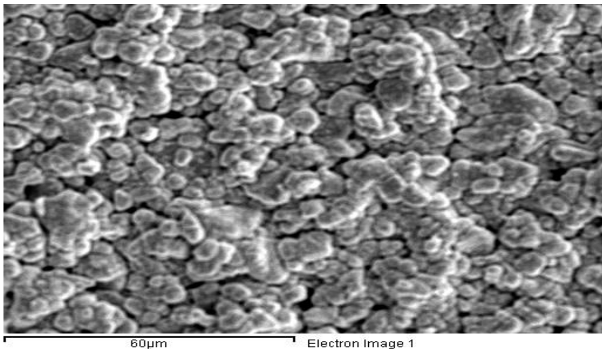
Figure 4 : Image MEB d'un échantillon de la 6 ème série, après traitement au \text{CdCl}_2 dans une solution saturée de méthanol
