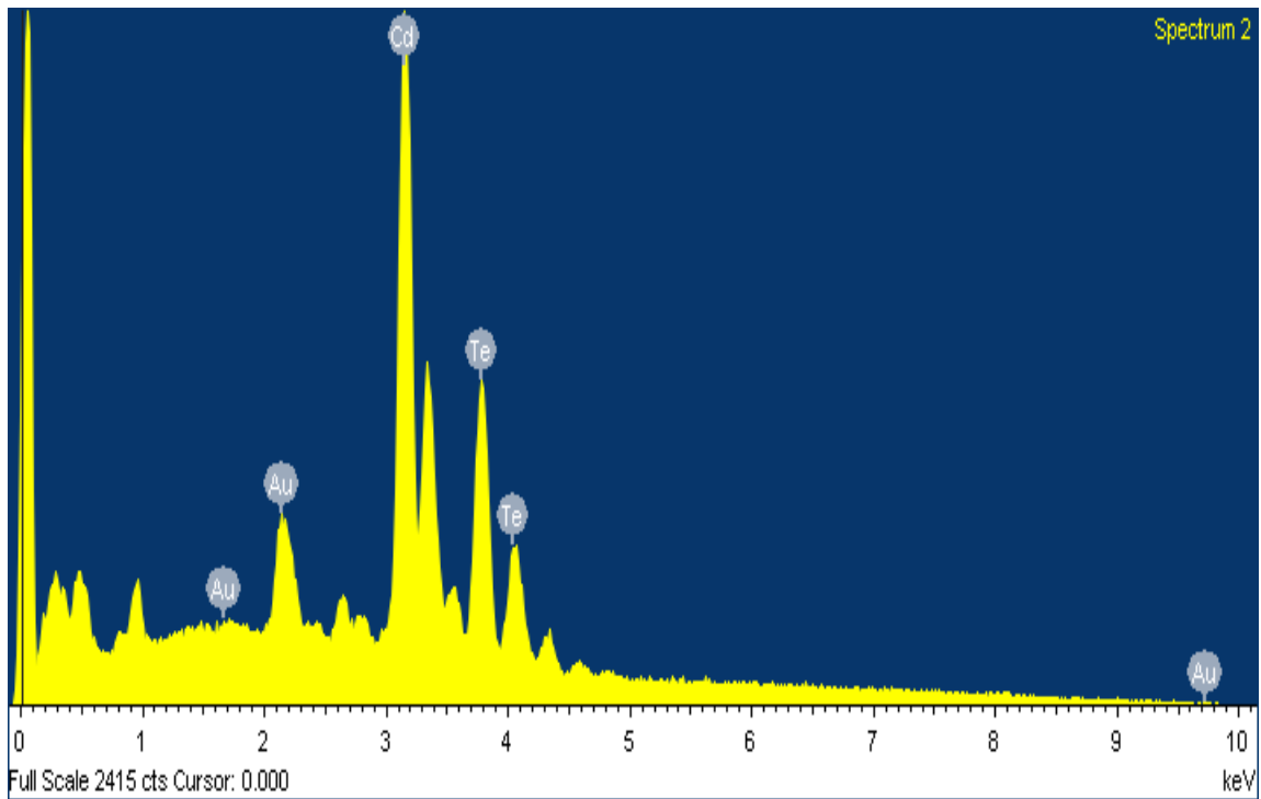
Figure 2 : Spectre EDS typique d'un film CdTe de la 11 ème série
