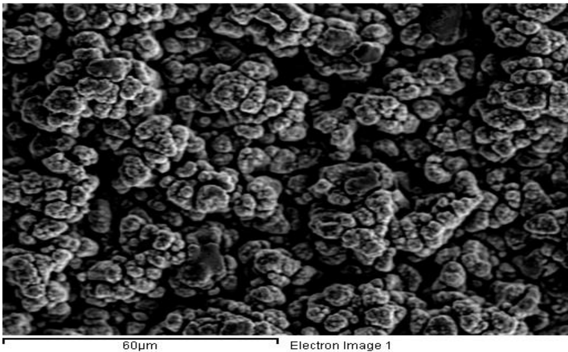
Figure 3 : Image du MEB d'un échantillon de la 6 ème série
