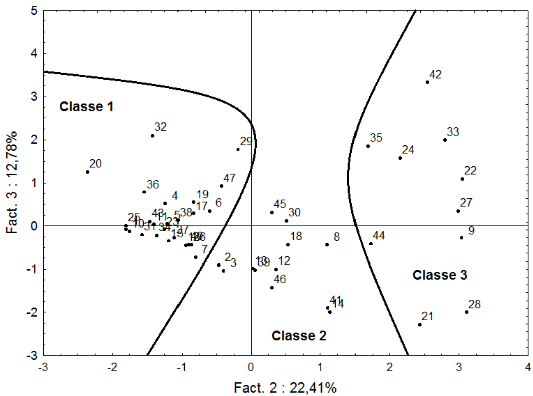
b) Analyse des US dans le plan factoriel F2-F3
