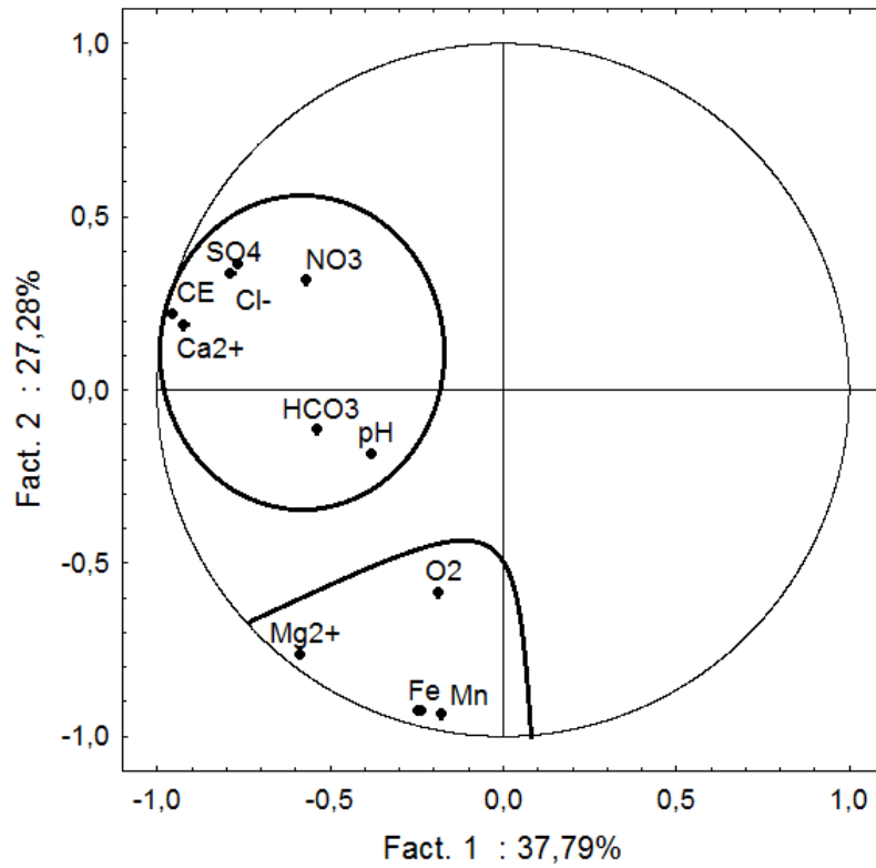
a) Analyse dans le plan factoriel F1-F2
