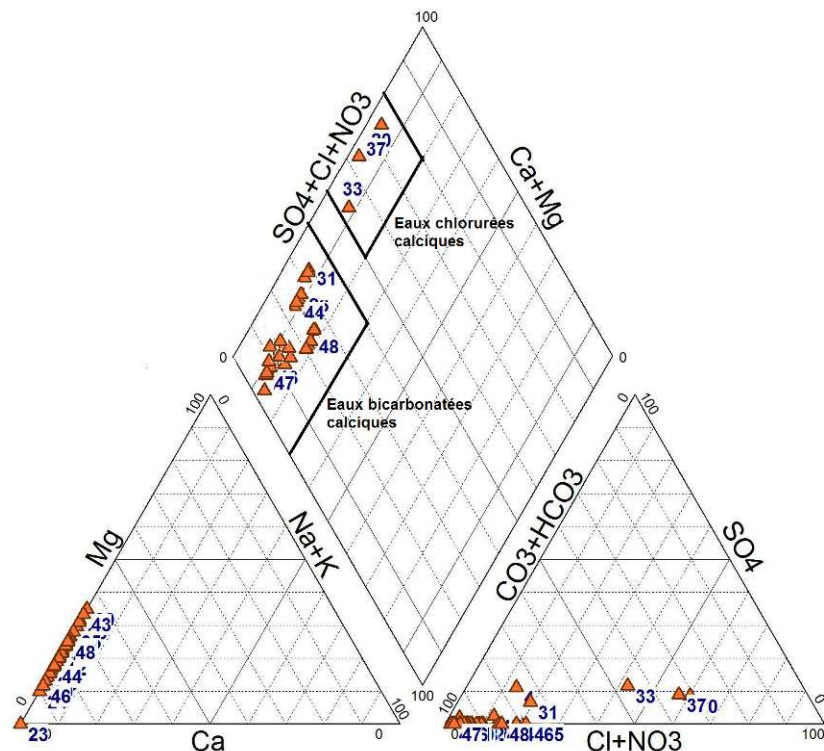
Figure 5 : Classification des eaux à l'aide du diagramme de Piper
