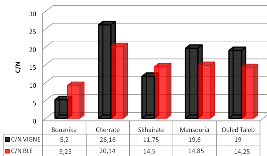
Figure 4 : Indice de fertilité des sols étudiés
