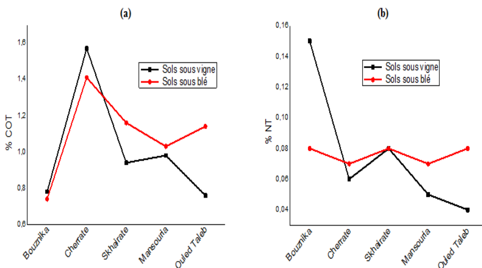
Figure 3 : Variation du carbone organique totale et azote total selon les stations
