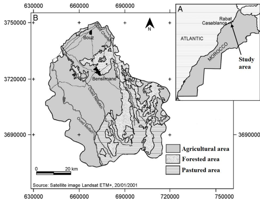
Figure 1 : Situation géographique de la zone d'étude
