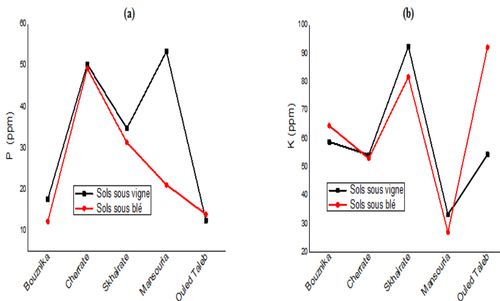
Figure 5 : Variation du phosphore et potassium selon les stations
