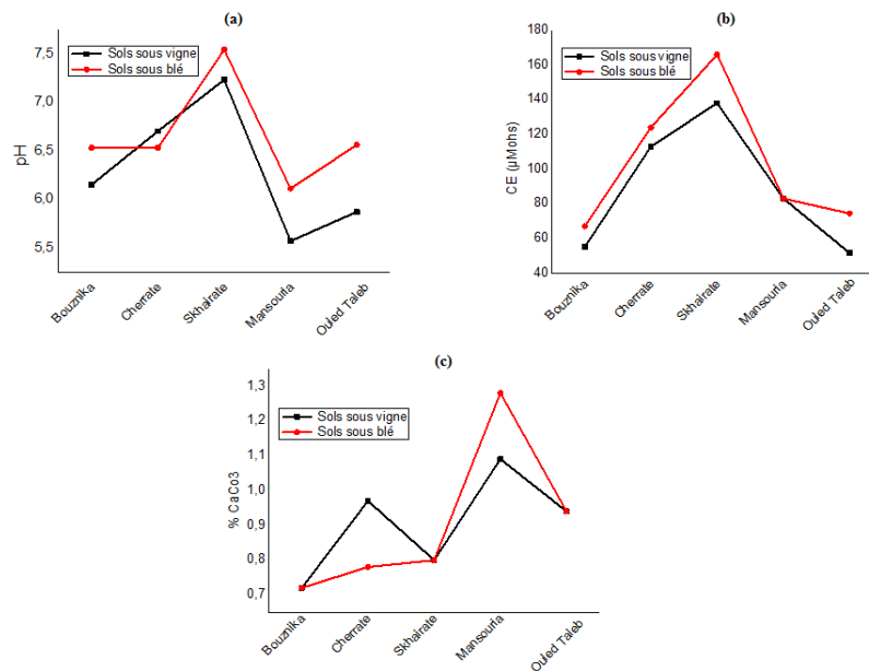
Figure 2 : Variation du pH, \text{CaCO}_3 et CE, selon les stations
