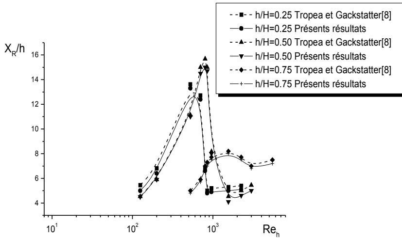
Figure 6 : La longueur de réattachement en fonction du nombre de Reynolds pour un obstacle rectangulaire (Incertitude pour Re_h : \pm 3\% et X_R/h : \pm 4.5\% )
